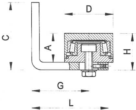
BOTTOM HINGE
